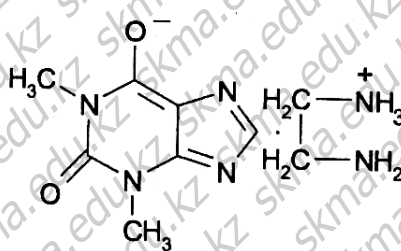
Эуфиллин – Euphillinum.
