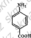
п-аминобензойная кислота
