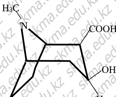
Эггонин
