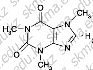
Кофеин-Coffeinum. 1,3,7-Триметилксантин.
