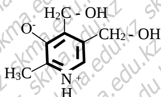
Цвиттер-ион
