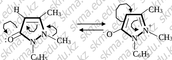
Цвиттер-ион (бетаин)
