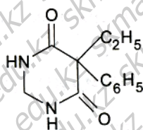
Гексамидин
