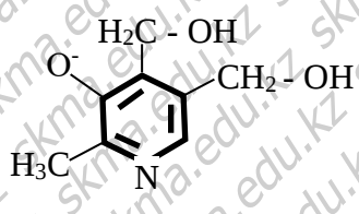
Фенолят
