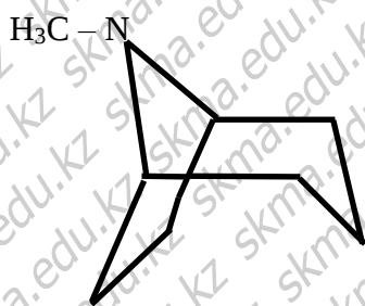
Тропан
