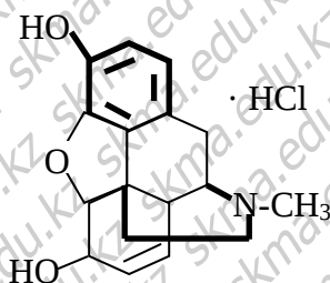
Морфин гидрохлориді
