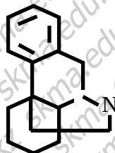
Морфинан
