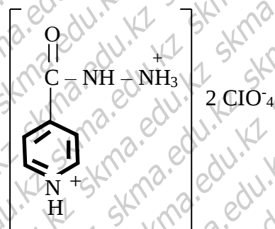
Изониазидтің липехлораты
